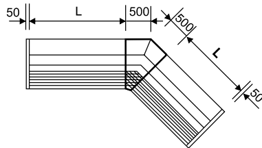
3) Open corner 135°
